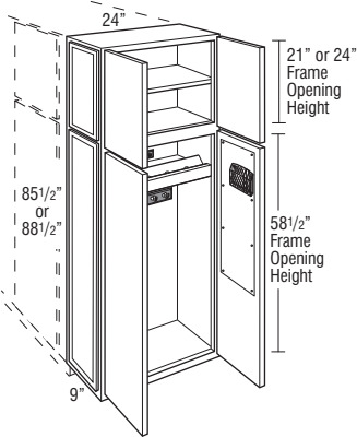
UOCDZ24909AEL/AER UOCDZ24939AEL/AER
